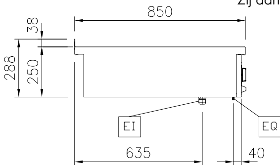
Zij aanzicht
