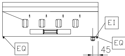
Front aanzicht
